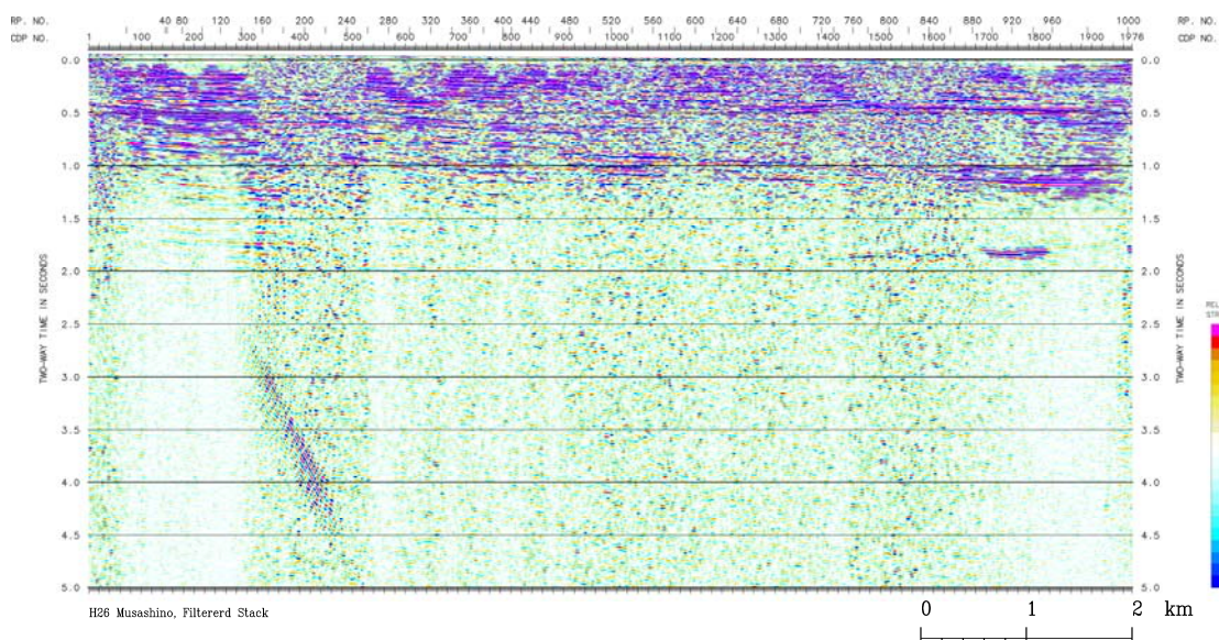
CMP 重合時間断面図。縦軸は往復走時 (秒)。
