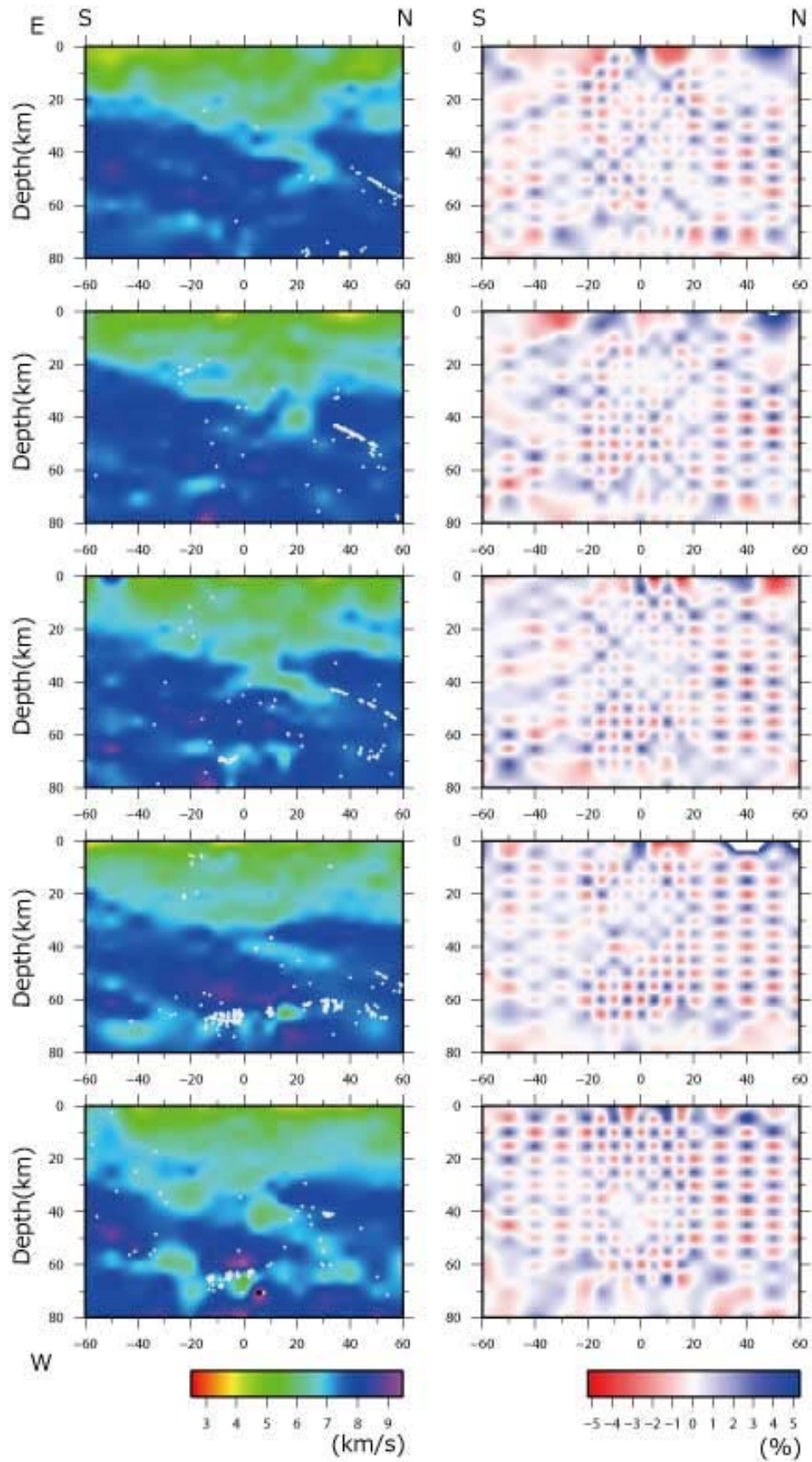
P波速度構造（南北断面）。左図：P波速度、右図：チェッカーボードテストの結果。上から順に東から西へ向かっての断面図が並んでいる。
