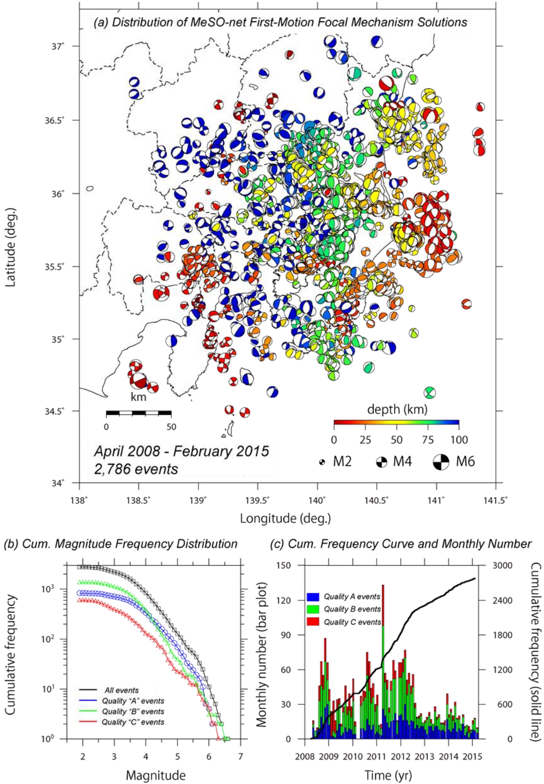
(a) 本課題において決定・整理した発震機構解の分布 (2008年4月1日~2015年2月9日)。色は震源の深さを表す。(b) 発震機構解の規模別頻度分布。(c) 発震機構解の一月当たりの決定数(棒グラフ)ならびに累積頻度曲線(黒線)。
