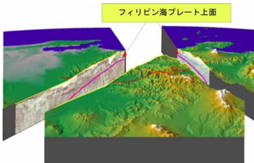
図 1. 2003 関東山地東縁測線と小田原-甲府測線のブロックダイアグラム。 二つの測線を繋ぐ赤い実線区間（飯能-御坂測線）で 2008 年に稠密地震観測を行った。
