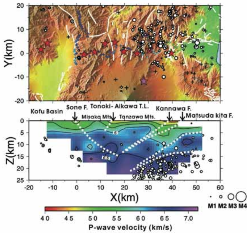
図4. 2005年小田原-山梨測線沿いの自然地震波トモグラフィー解析によるP波速度構造 (蔵下ほか, 2009)
