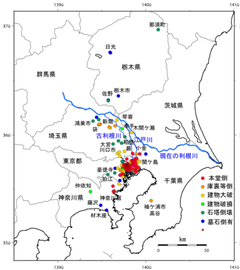
(左) 1855年安政江戸地震による関東地方の寺院被害
