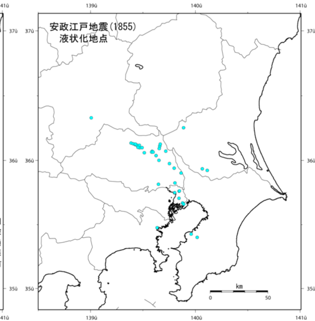
(右) 同地震による液状化発生地点
