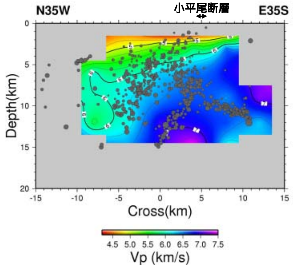
上図. 推定されたP波速度構造と震源分布を示す。
