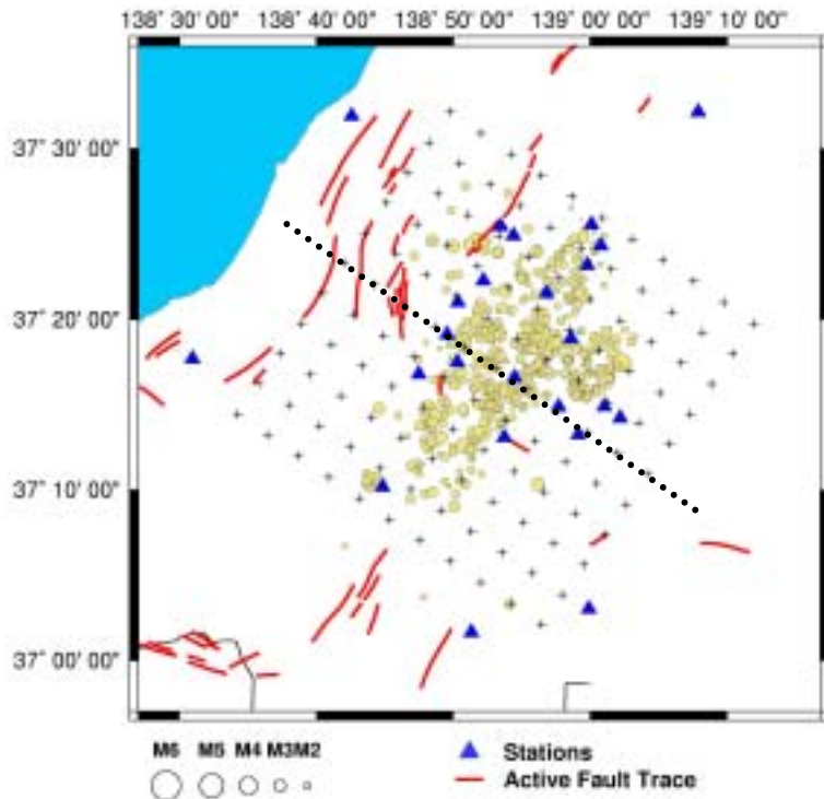
左図. 使用したグリッド配置、観測点分布、求めた震源の震央分布を示す。点線は上図の断面図の位置を示す。
