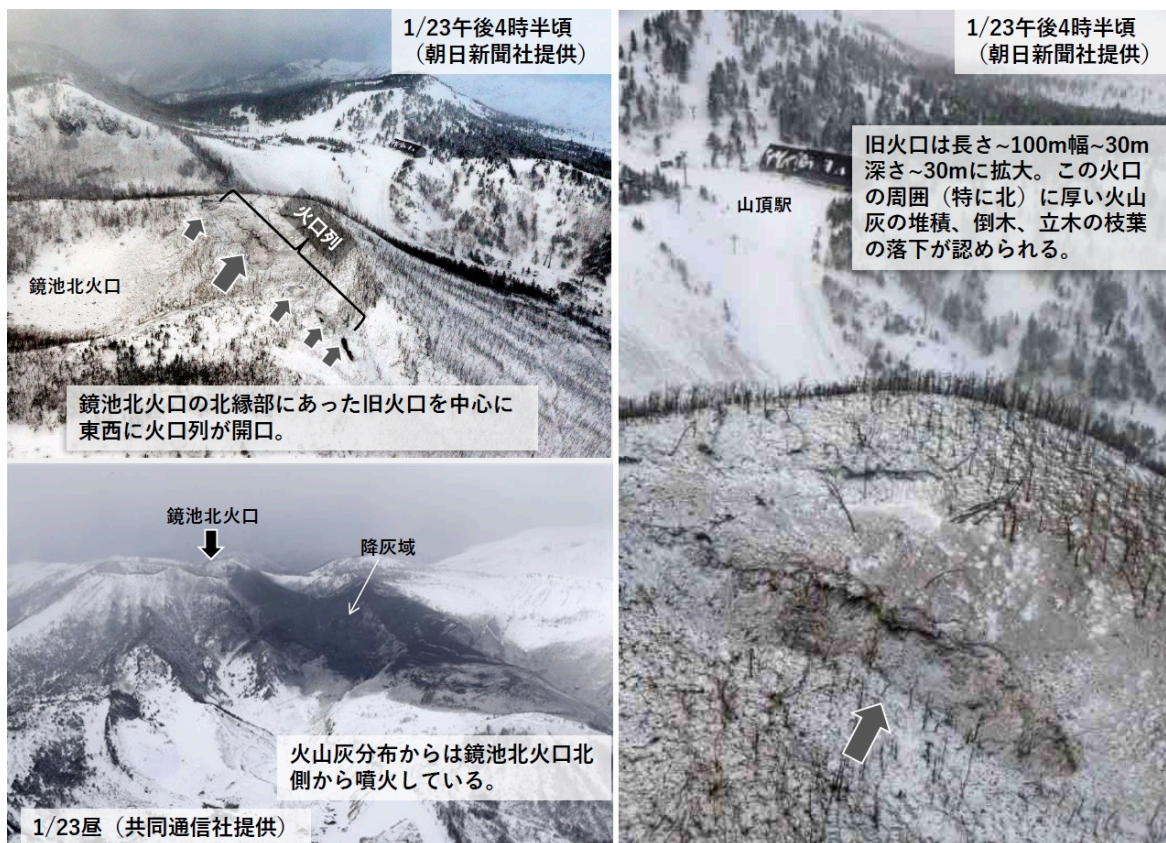
図2 1月23日噴火の火口域や降灰範囲を示す写真
