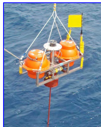
堆積物中の温度を長期計測する装置
