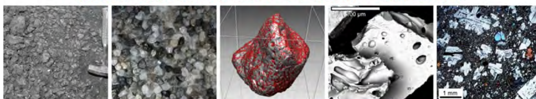
構成物・粒子物性の解析, 岩石微細構造・鉱物組成・組織の分析
