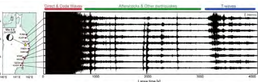
2008年岩手県沿岸北部の地震時に観測されたT相。東北地方の太平洋側の沿岸部で海中音波に変換し、天皇海山列にぶつかり反射・散乱されてきたT相が陸域の地震計で観測された。 (Obara & Maeda 2009)
