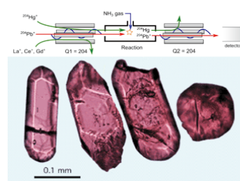
ジルコンの超高精度同位体分析
