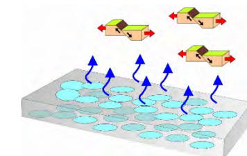
いわき地域群発地震の概念図
