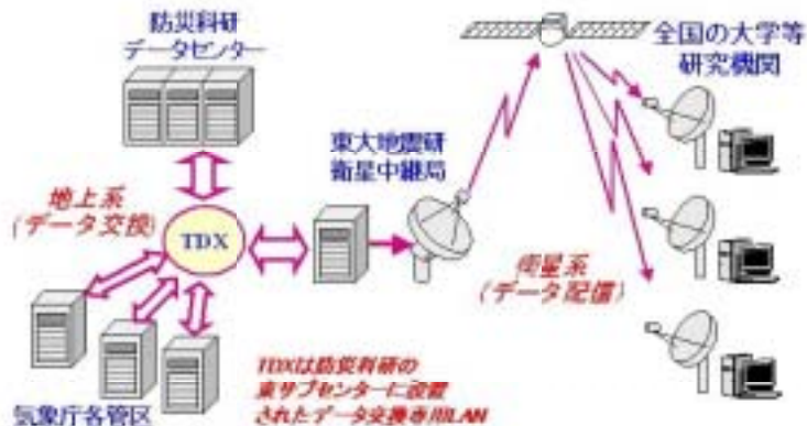
図1 高感度地震波形データの全国リアルタイム流通システム
