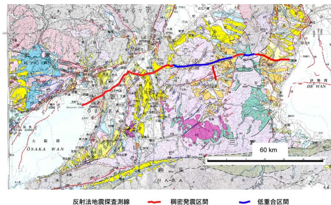
図1 近畿横断地殻構造探査測線図。基図は、水野ほか1)による。
