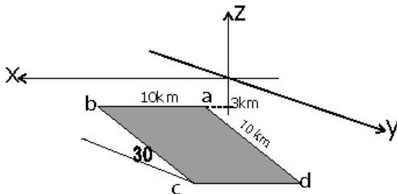
図 1：シミュレーションに用いた仮想的な断層.
