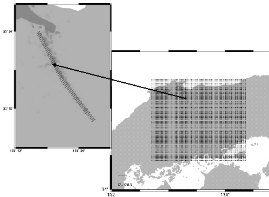
図 6：鳥取県西部地震の断層形状（Wu et al., 2000 5) ）（左）と地表の領域（右）
