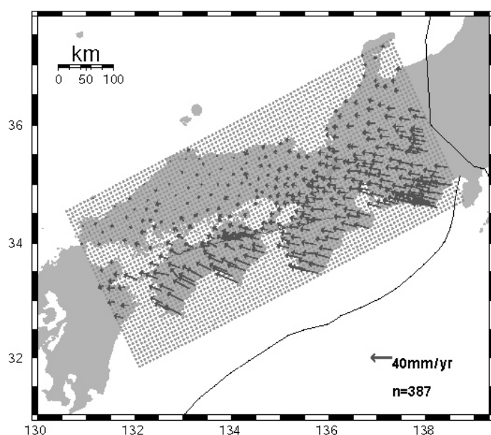
図 3：西南日本の GEONET による GPS 変位速度場。
