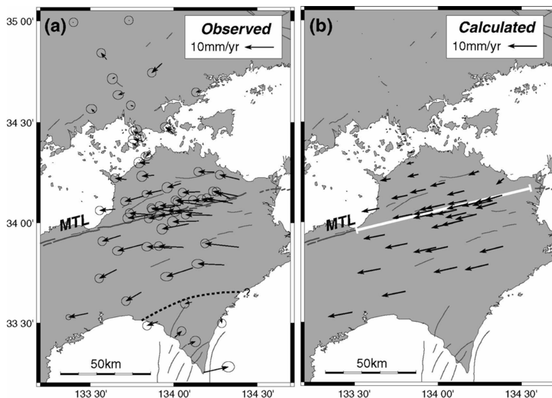
図3 (a)弾性圧縮変形を除去した残差速度場。南海トラフの地震サイクルに関与しない永久変動を表す。(b)中央構造線の最適モデルから計算した前弧のブロック運動。最適モデルのパラメータ値は、断層面傾斜角 35^\circ 、上部固着域の深さ 15km、深部すべり速度 9mm/yr である。
