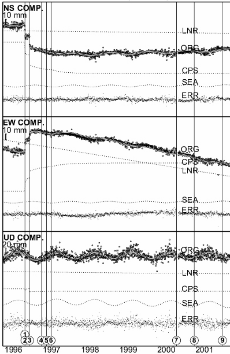
図1．GEONET 観測局の座標成分の時系列の例。上から、南北、東西および上下成分で、ORG が観測データ、LNR が直線トレンド、CPS が地震時＋余効変動、SEA が年周変動、ERR がモデル化できない誤差である。
