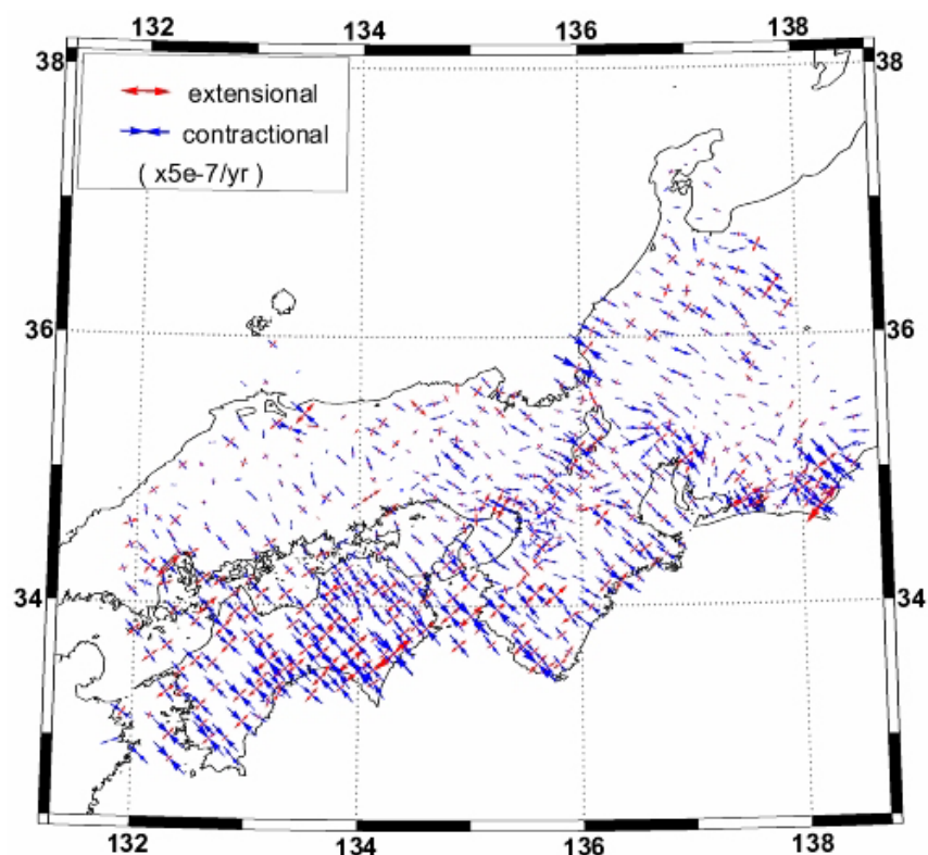
図 4. 中部～近畿～中四国の GEONET 観測データから推定した 1996 年から 2002 年までの歪速度の主軸の分布
