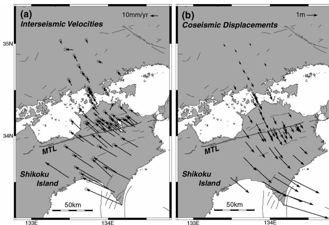
図2 (a)稠密 GPS 観測による地殻水平速度。アムール・プレートに対する速度を表す。(b) Sagiya and Thatcher (1999) 3) のモデルを用いて計算した 1946 年南海地震の際の地殻変動。
