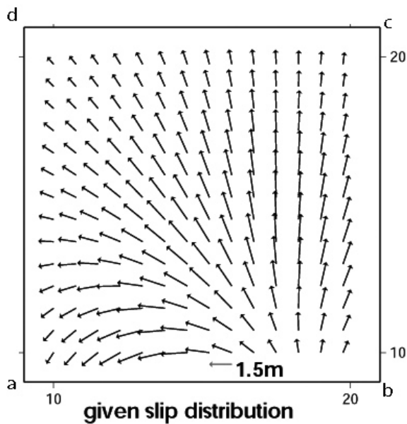
図 2：仮想断層面上に与えた仮想スリップ分布。 縦横軸の単位：km
