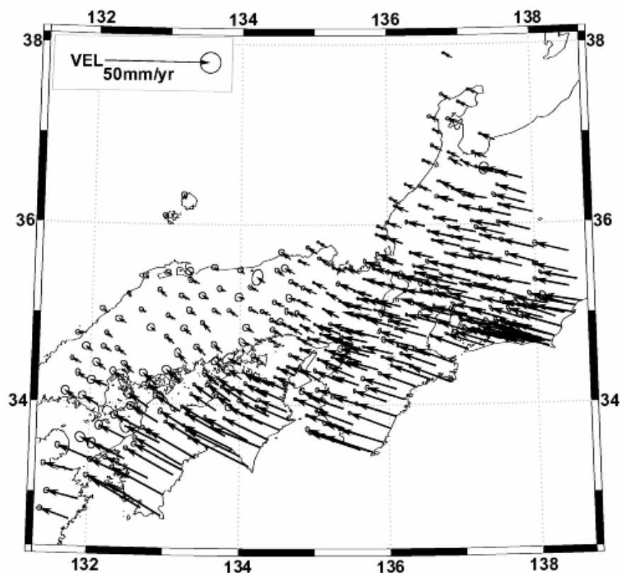
図 3. 中部～近畿～中四国の GEONET 観測データから推定した 1996 年から 2002 年までのアムール・プレートに対する水平速度分布
