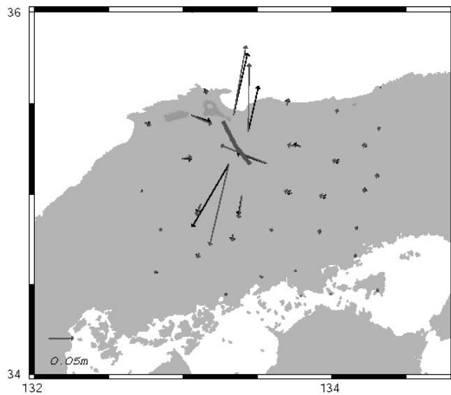
図 7 : GPS と水準データから推定された鳥取県西部地震の断層面上のすべり分布 (上) と GPS 観測点での観測値と計算値の比較 (下)。
