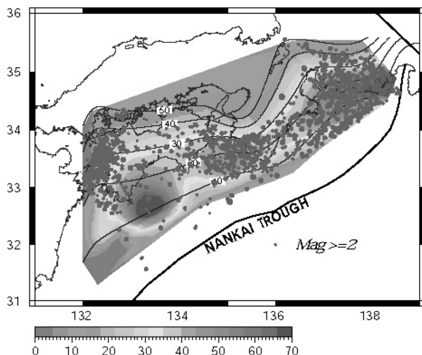
図4：推定された固着率分布．M2以上の地震の震源も示す．
