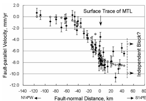
図4 中央構造線に直交する線上に投影した、断層に平行な速度成分のプロファイル。
