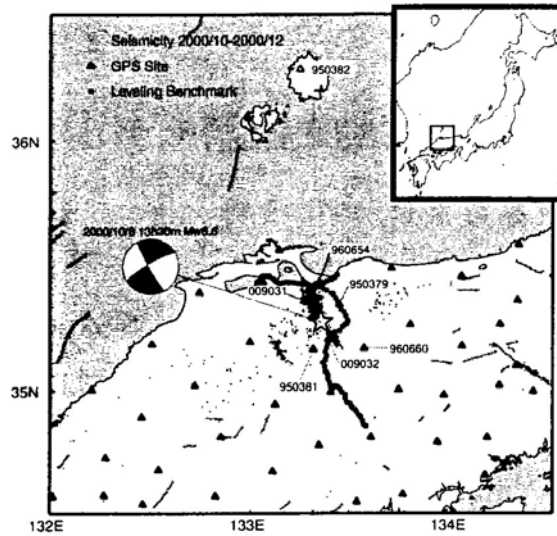
図 5：2000 年鳥取県西部地震のメカニズム，余震分布と GEONET 水準点（鷺谷他，2002 4) より）
