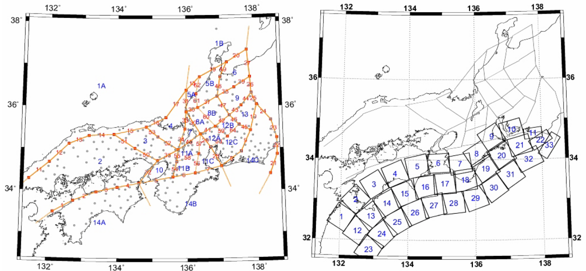
図 2. 中部～近畿～中四国のブロックおよび断層のモデル
