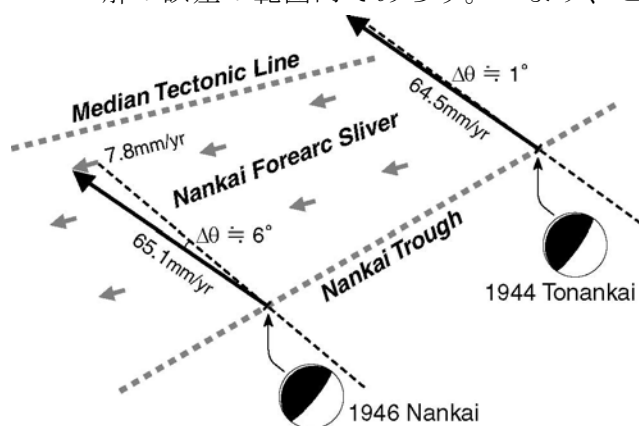
図 1 南海トラフにおける地震のメカニズムとプレート相対運動ベクトルとの関係。南海地震の領域では地震のスリップベクトルとプレート運動の方向が一致せず、地震と地震の間に前弧ブロックが定常的横すべり運動をしていることを予想させる。
