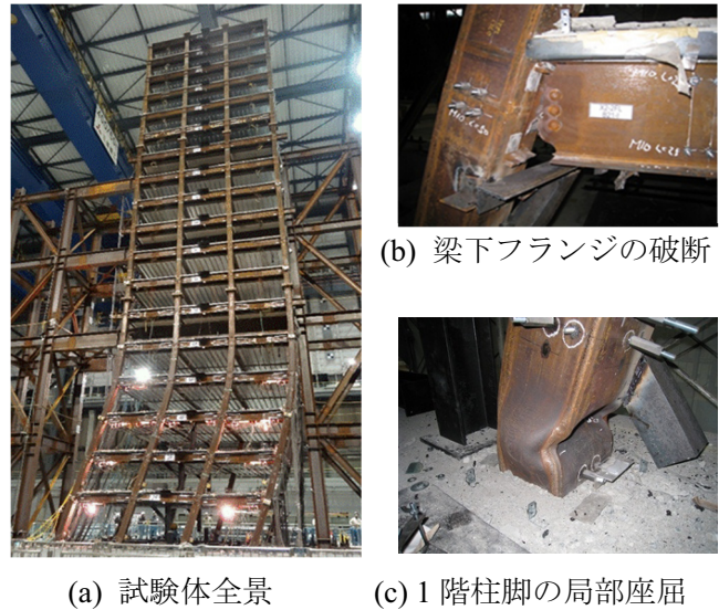
図3 E-ディフェンス振動台実験での崩壊挙動
