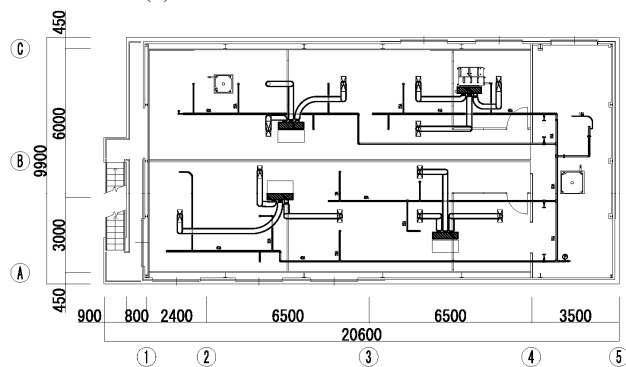
(b) 設備の配置図
