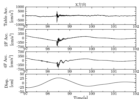
図 18 擁壁衝突時拡大波形（免震2 X 方向）
