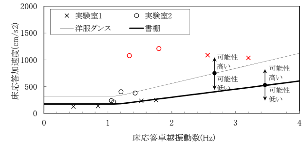
図 52 家具の転倒可能性 (赤印は JMA 神戸 75%)
