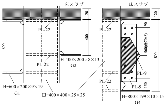
(a) 桁行方向 中柱 A, B 通り (b) 梁間方向 1, 3 通り
