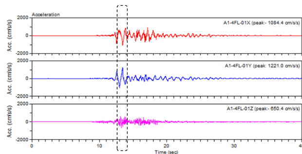
(d) 実験室 2 の床応答加速度
