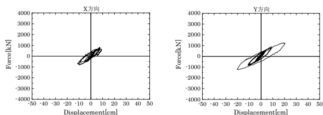
X 方向 Y 方向 図 12 免震 1 免震層変位と層せん断力の履歴（JMA 神戸波 80%）
