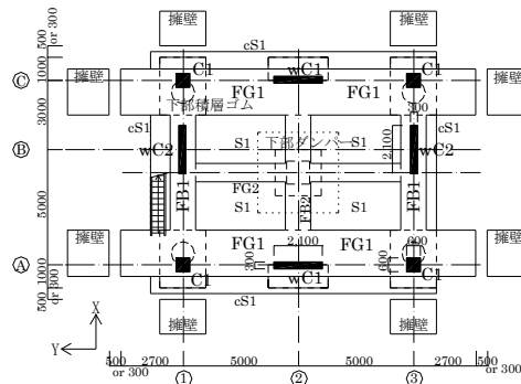
1階床伏図
