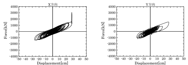
X 方向 Y 方向 図 16 免震 2 免震層変位と層せん断力の履歴 （三の丸波）
