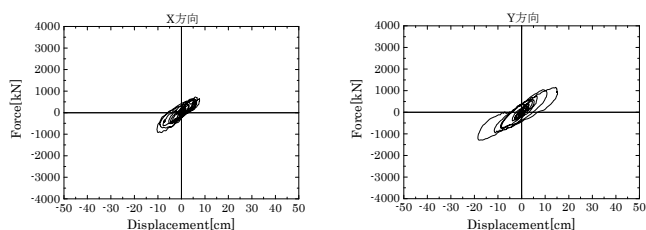
X 方向 Y 方向 図 13 免震 2 免震層変位と層せん断力の履歴（JMA 神戸波 80%）
