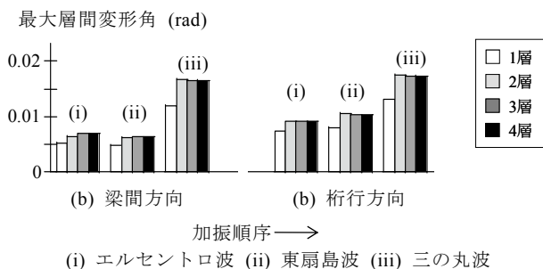
図 13 各加振に対する最大層間変形角
