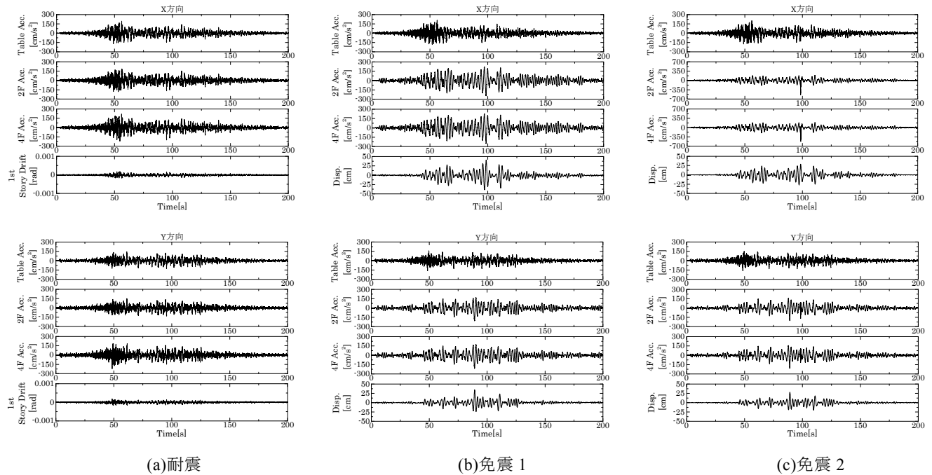
図 14 三の丸波による応答時刻歴波形（上図：X 方向、下図：Y 方向）
