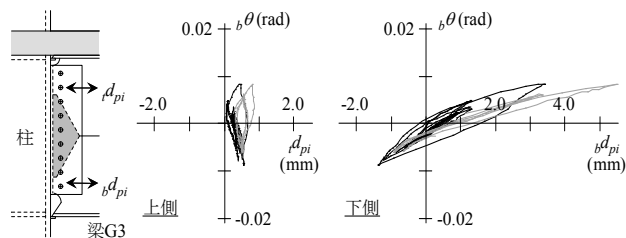
図 15 現場溶接接合部の梁端ウェブとシャーププレートのボルト接合部におけるすべり性状（三の丸波加振時）
