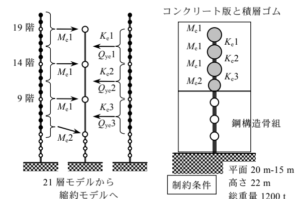
図2 骨組実験システム用モデル
