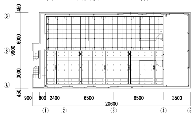
(a) 天井伏図と間仕切り壁の位置
