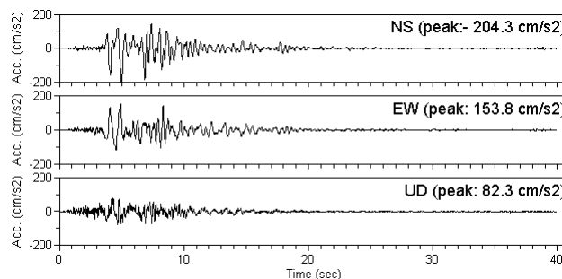
(c) JMA 神戸観測波 本震 25%
