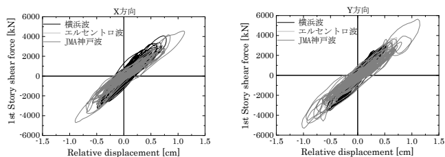
X 方向 Y 方向 図10 層間変位と層せん断力の履歴
