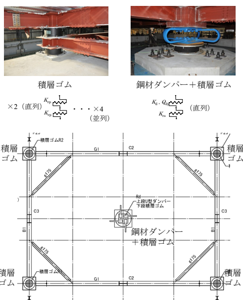
図 36 縮約層 2 の詳細
