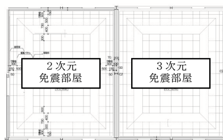
(b) 平面図
