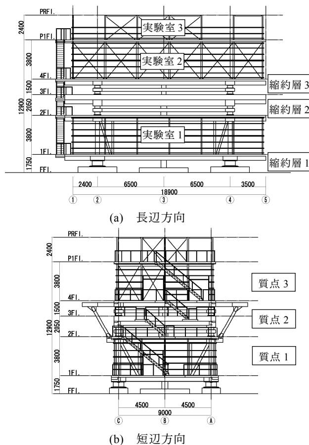
図 35 室内実験システムの立面図
