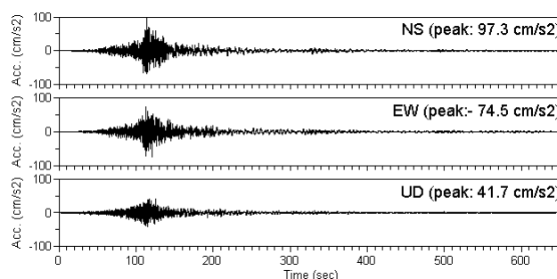
(a) 西新宿観測波 本震 100%
