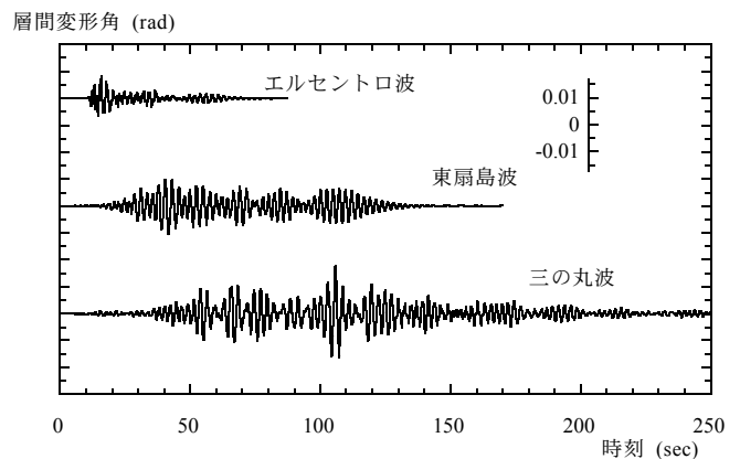
図 11 骨組の 2 階に生じた層間変形角の時刻歴波形
