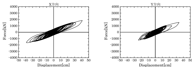
X 方向 Y 方向 図 15 免震 1 免震層変位と層せん断力の履歴 （三の丸波）
