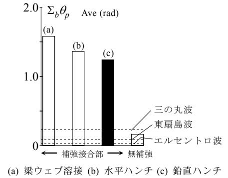
図 23 補強による変形能力の向上
