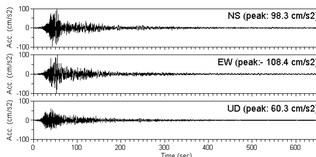
(b) 西新宿観測波 余震 330%
