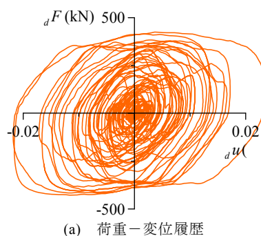
図 29 三の丸波加振時におけるオイルダンパーの応答
