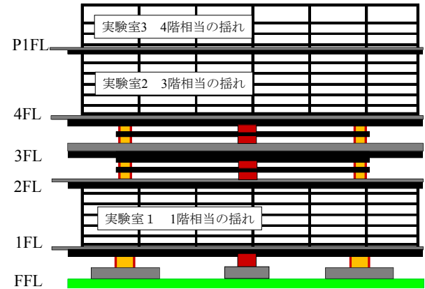
図 50 超高層建物実験で再現される揺れ
