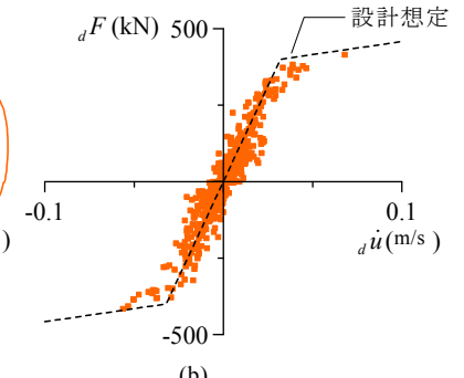
図 29 三の丸波加振時におけるオイルダンパーの応答
