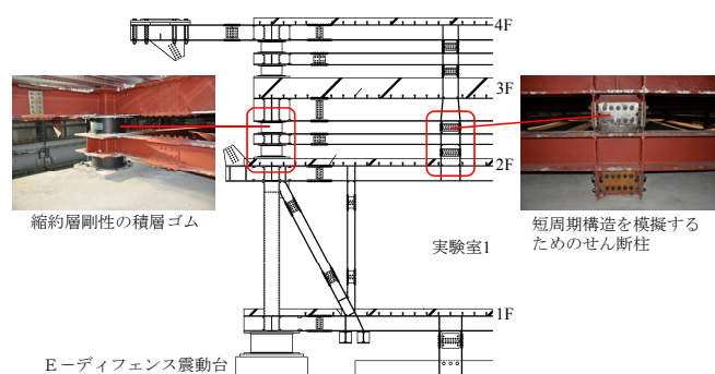
図 37 縮約層部分の詳細
