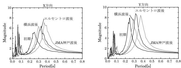
X 方向 Y 方向 図9 耐震構造の応答倍率 (固有周期の変化)
