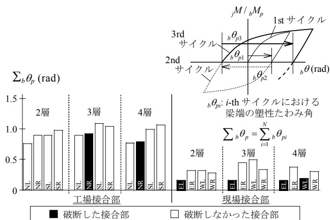
図 17 累積塑性回転角に基づく変形性能評価
