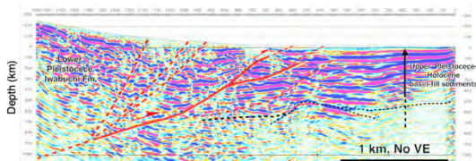
富士川河口断層帯・入山瀬断層の高分解能イメージング
