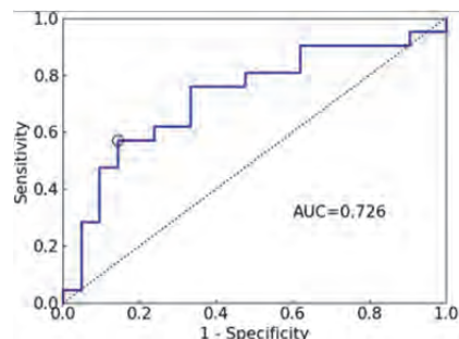
桜島の活動的の火口近傍のミュオグラフィデータセットに対する ROC 曲線。(Nomura et al. Sci Rep. (2020))
