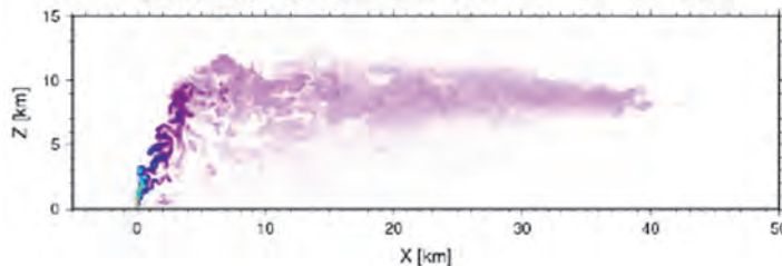
火山噴煙の3次元シミュレーション
