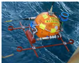
開発した自由落下自己浮上式海底地震計
