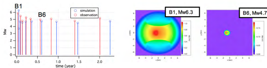
東北沖地震後のマグニチュードの時系列。
