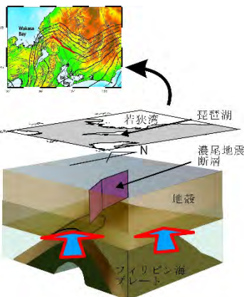
濃尾地震発生域の構造の概念図
