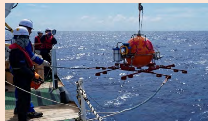
太平洋アレイ計画での機器設置
