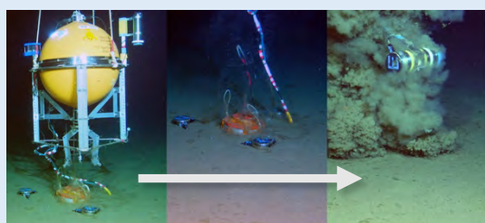
深海での回収時の動作を無人潜水艇で確認
