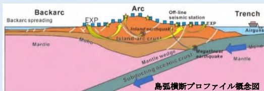
島弧横断プロファイル概念図
