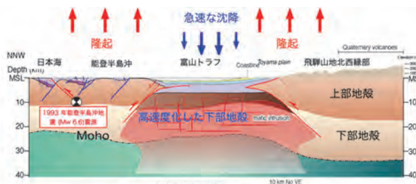
中新世リフト帯の再活動による能登半島・富山トラフの第四紀テクトニクス
