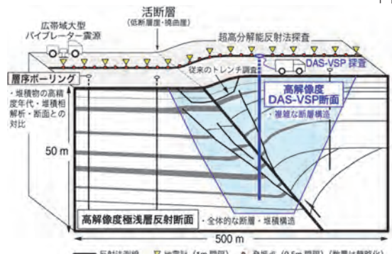
DAS-VSP による Seismic trench 法の開発
