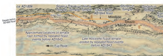
古絵図の地理情報解読と現在の地形の比較による 1854 年安政東海地震に伴う富士川河口の地形変化
