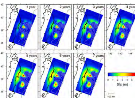
2011年東北沖地震後7年間の余効すべりの時間発展
