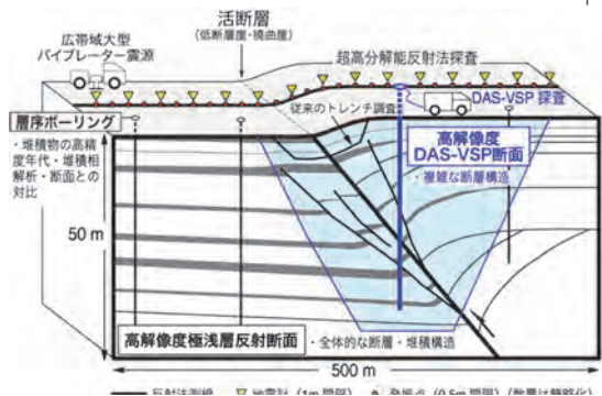
DAS-VSP による Seismic trench 法の開発
