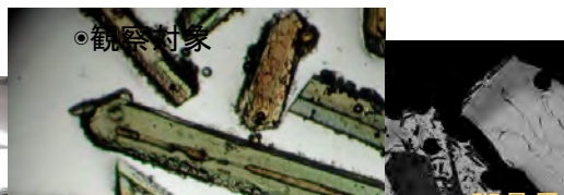
斑晶累帯構造
