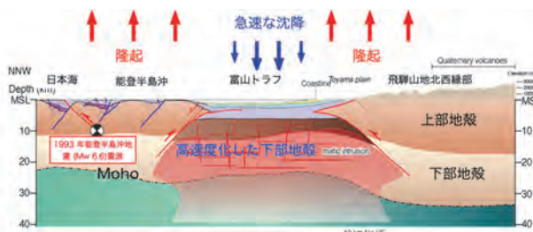
中新世リフト帯の再活動による能登半島・富山トラフの第四紀テクトニクス
