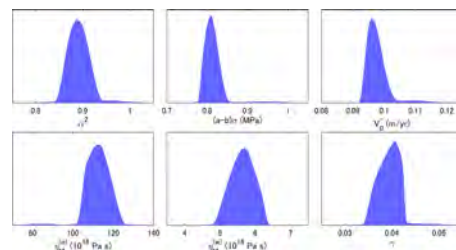
測地データを用いた数値モデルのパラメータ推定
