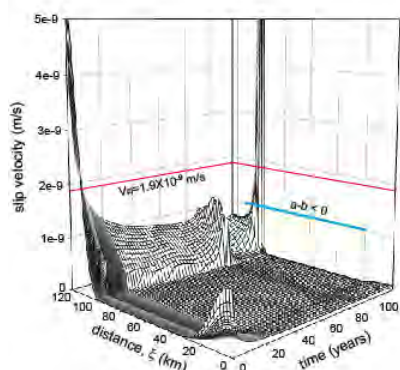
図1. 沈み込み域のプレート境界地震発生の数値シミュレーション結果。地震発生に至るまでの断層すべりの時空間発展を示す。すべり速度をプレート境界に沿って測った距離(地表は \xi=0 )と前の地震からの経過時間の関数として示している。
