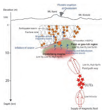
箱根火山のマグマ供給モデル
