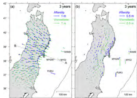
2011年東北沖地震後3年間の余効すべりと粘弾性緩和による地殻変動
